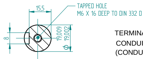
Przekrój A-A 1:1
